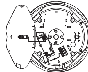
Tilkobling sensor
