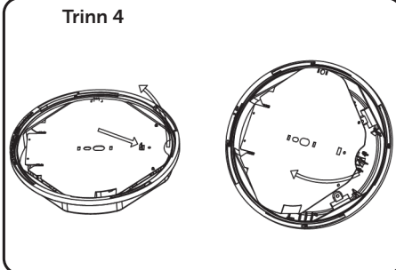
Trinn 4
