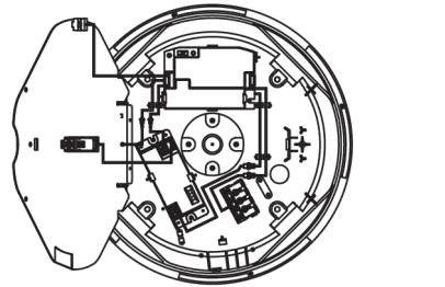
Tilkobling Sensor + Nødlys-KIT
