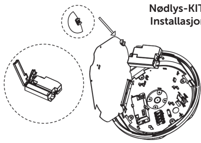
Tilkobling Sensor + Nødlys-KIT
